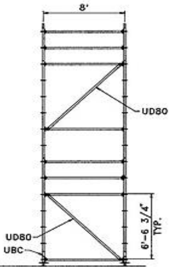
END ELEVATION
